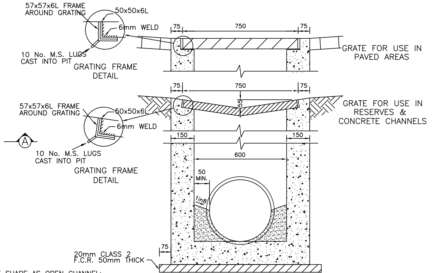
SECTION A-A
